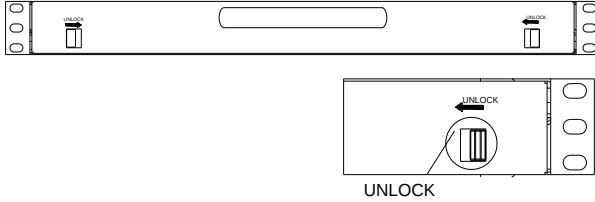
图 2-3 解锁方式
